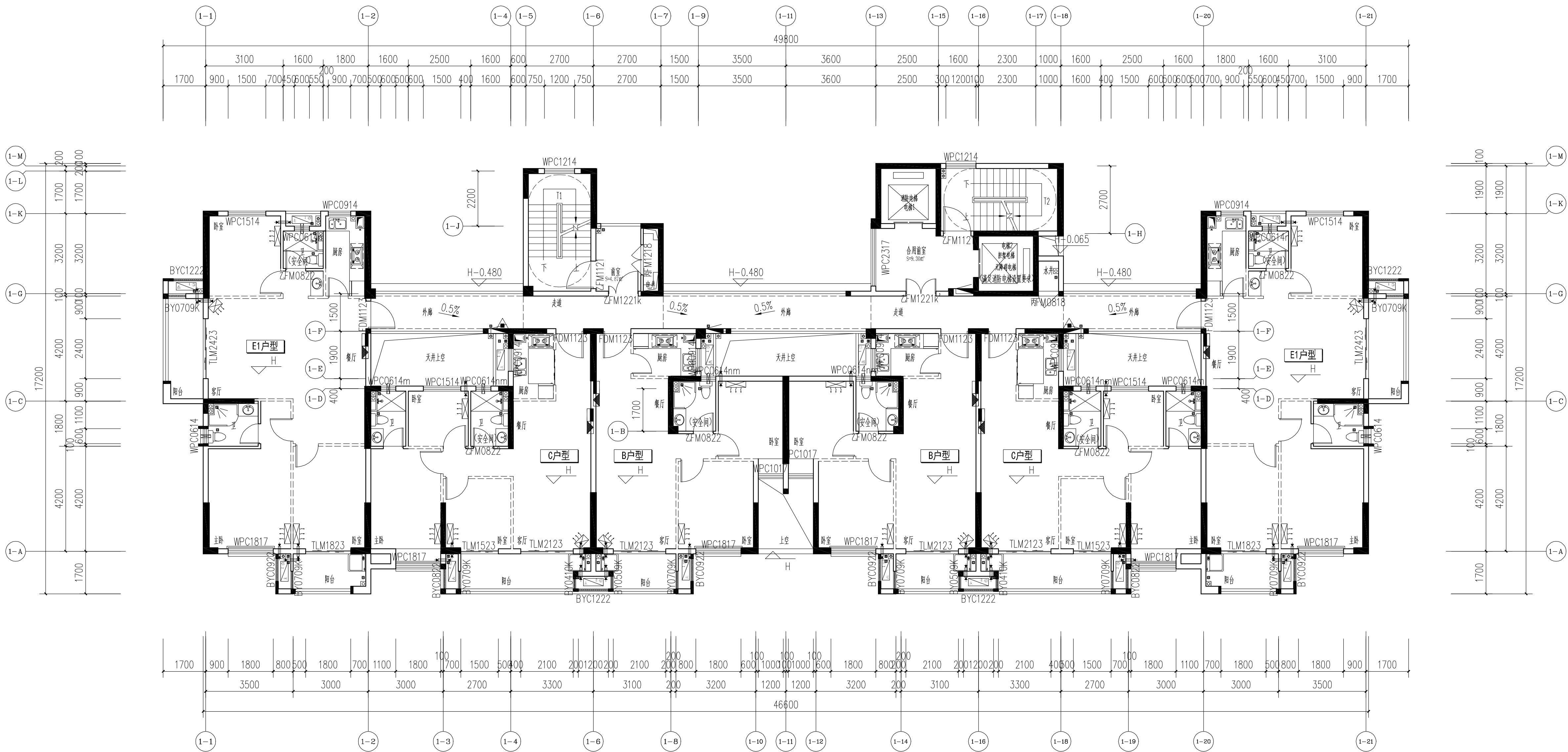
1#楼二~十九层平面图
